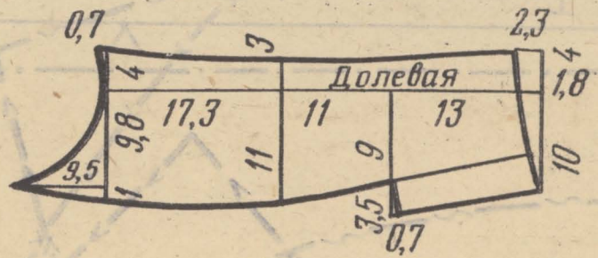
Нижняя половинка рукава. 2 дет.
