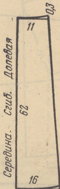
Заднее полотно юбки 1 дет.
