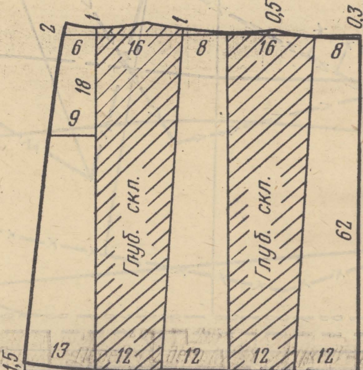
Переднее полотно юбки 1 дет.
