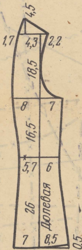
Заднее полотно юбки 1 дет.
